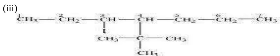
4-Tert-Butyl-3-iodoheptane
