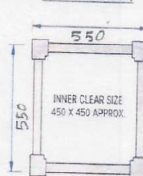
RCC PANEL (4 NOS.)
